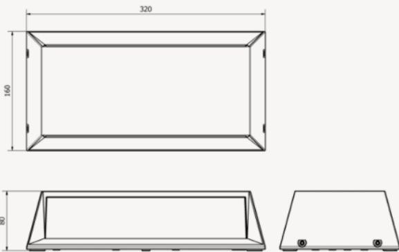
Schutzwanne SYMM Plus (Abmessungen in mm)
