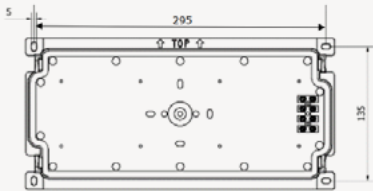
Montageplatte SYMM (Abmessungen in mm)
