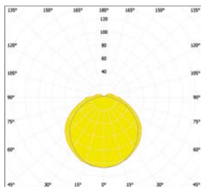
POLARDIAGRAMM TPN | OPAL
